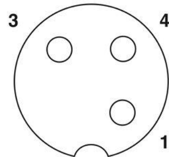
Polbild M12-Buchse, 3-polig, A-kodiert, Ansicht Buchsenseite
