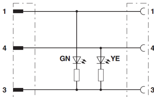
Schaltplan
