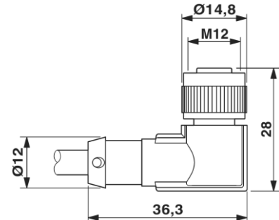
Buchse M12 x 1, gerade, mit LED
