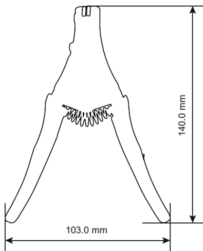
Abmessungen Zange
