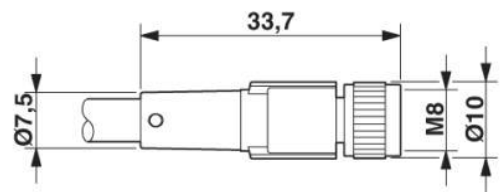
Buchse M8 x 1, gerade
