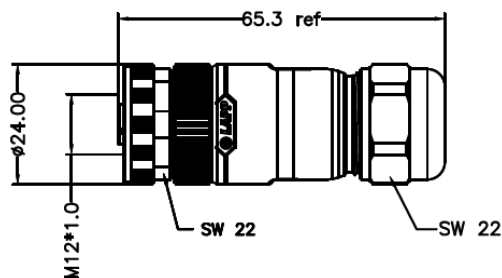
Technische Zeichnung
