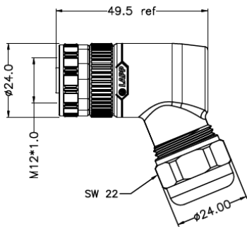
Technische Zeichnung
