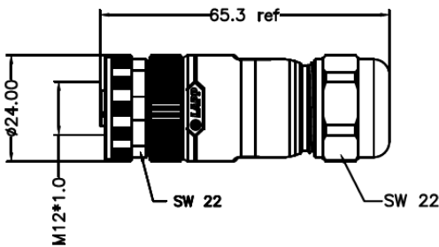
Technische Zeichnung
